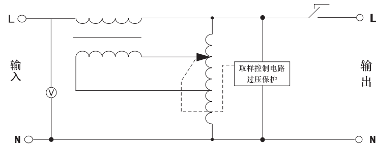
单相15kVA~30kVA电气原理图
