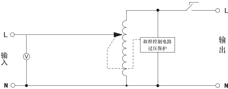
单相0.5kVA~10kVA电气原理图
